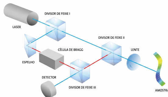
Figura 2: Vibrometria por Laser Doppler. Fonte: [5].
